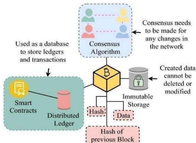
Gambar 1. Komponen Blockchain
